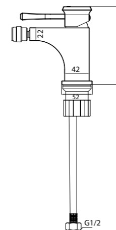
MIL-BD-CRM Смеситель для биде
