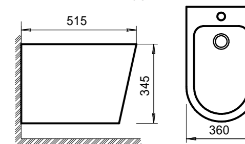
Биде подвесное BB053BH
