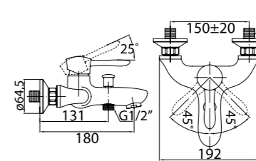
OGL-VAS-CRM Смеситель для ванны и душа
