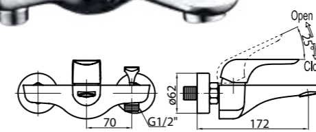
NOT-VASM-CRM Смеситель для ванны и душа
