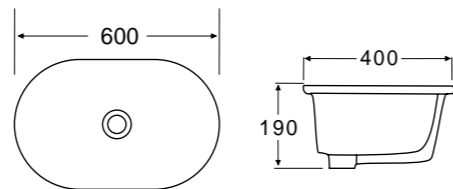
Раковина накладная new BB1004
