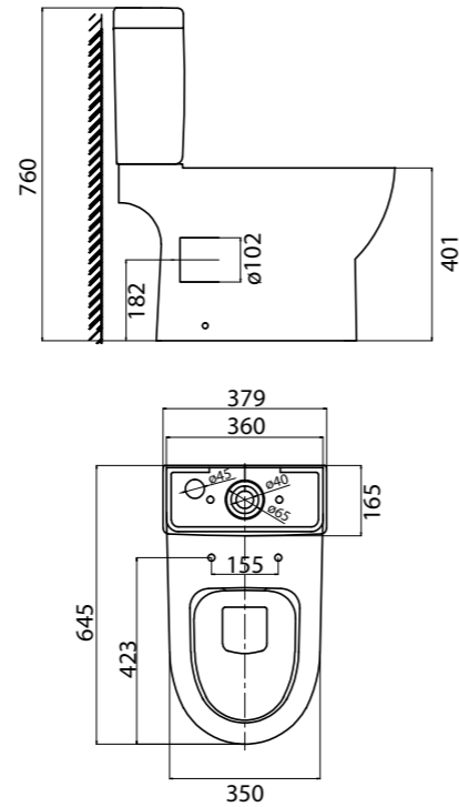
Унитаз компакт безободковый BB130CPR | BB130T | BB130SC Чаша унитаза | Бачок | Сидение
