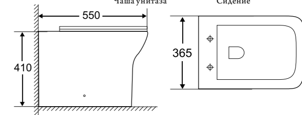
Унитаз приставной безбодковий BB248CBR | BB2112SC Чаша унитаза | Сидение
