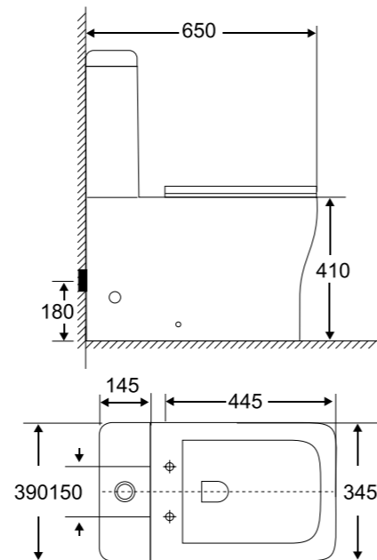
Унитаз компактный безбодковий BB248CPR-P | BB248T | BB2112SC Чаша унитаза | Бачок | Сидение
