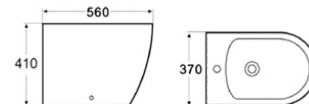
Биде BB2141B Биде
