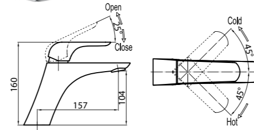
NOT-LVM-CRM-W0 Смеситель на раковину
