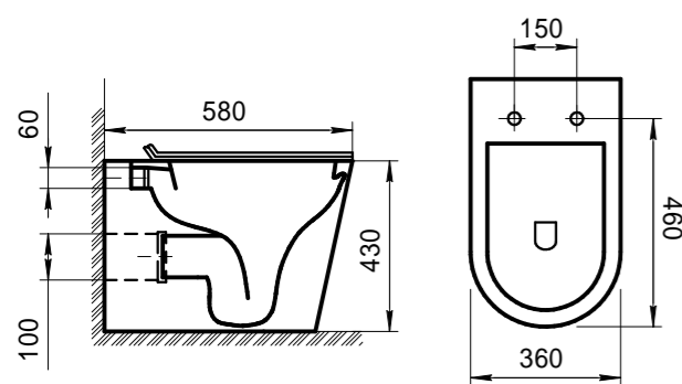
Унитаз приставной безободковый BB1003CBR | BB2111SC Чаша унитаза | Сидение
