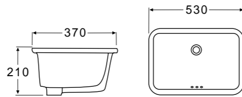
Раковина керамическая встраиваемая снизу NEW BB1006
