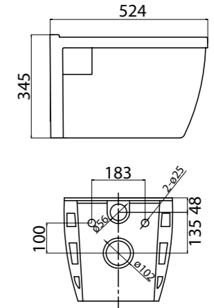
Унитаз подвесной безободковый BB070CHR | BB070SC Чаша унитаза | Сидение
