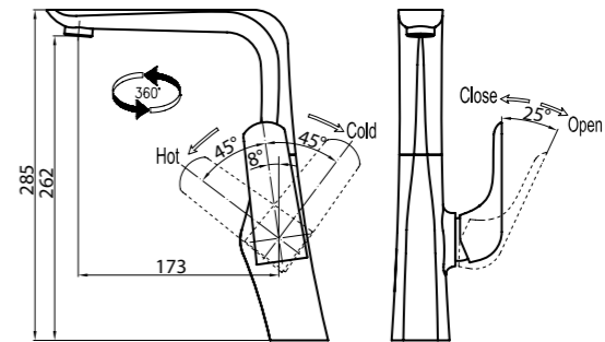
NOT-LAM-CRM Смеситель для кухни
