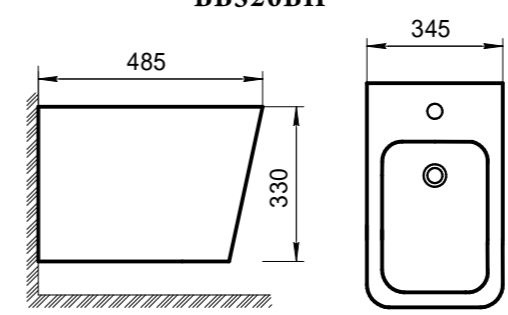
Биде подвесное BB520BH
