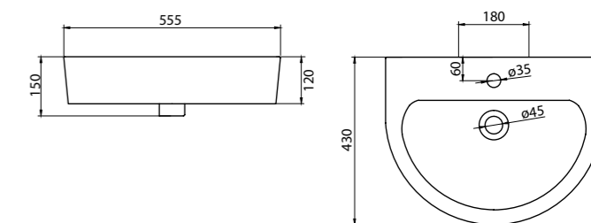
Раковина на пьедестале BB105L | BB105P Чаша раковины | Пьедестал
