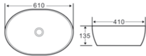
Раковина накладная BB1348
