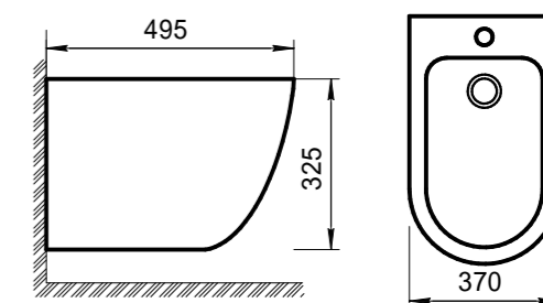
Биде подвесное BB046BH Биде
