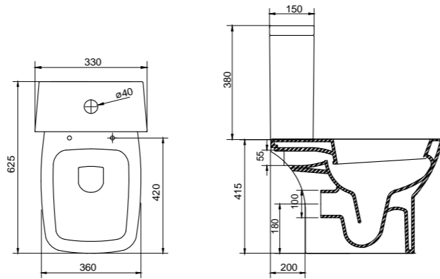
Унитаз компакт безбодковий BB128CP | BB128T | BB128SC Чаша унитаза | Бачок | Сиденье
